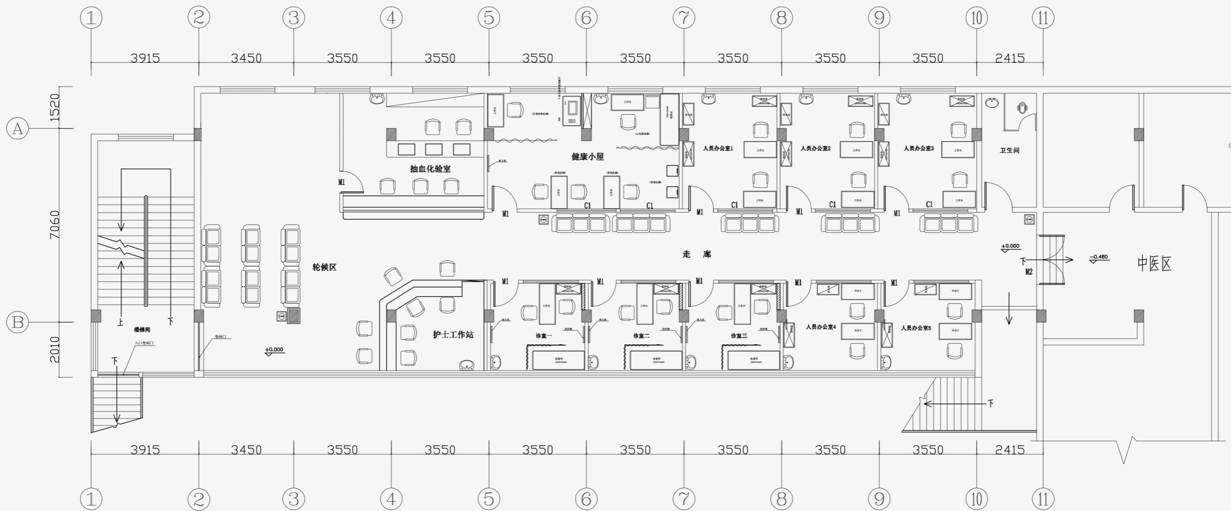
平面布置方案
